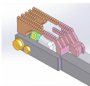
OP 前後差動送り機構
