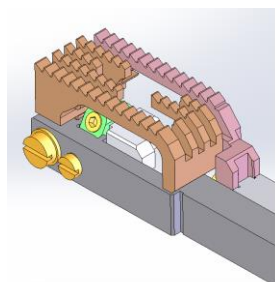
左右差動送り機構
